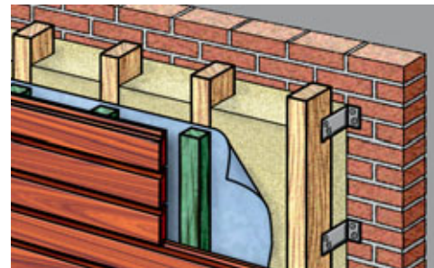
Opbouw gevelbekledingsconstructie bij een steenachtig binnenspouwblad, regelwerk verduurzaamd.
